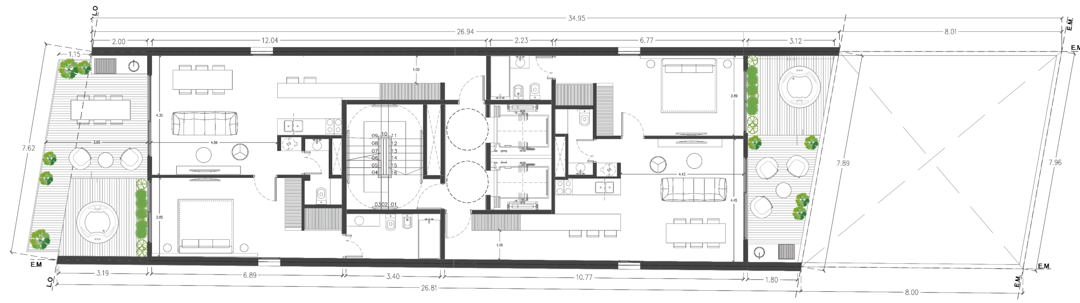
PLANTA 10°
