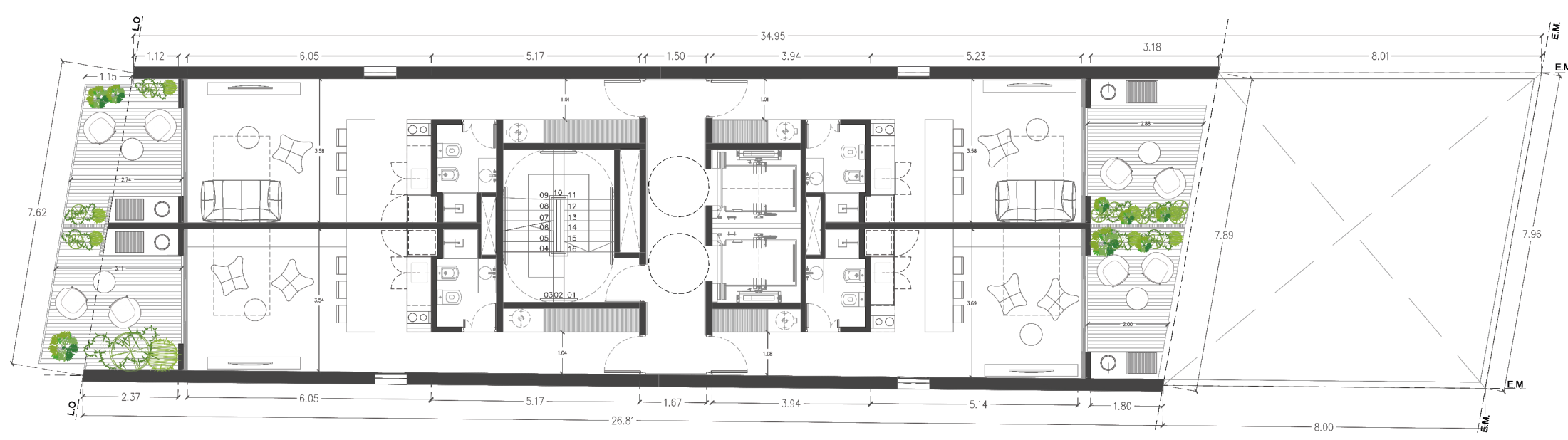
PLANTA TIPO 1°- 9°
