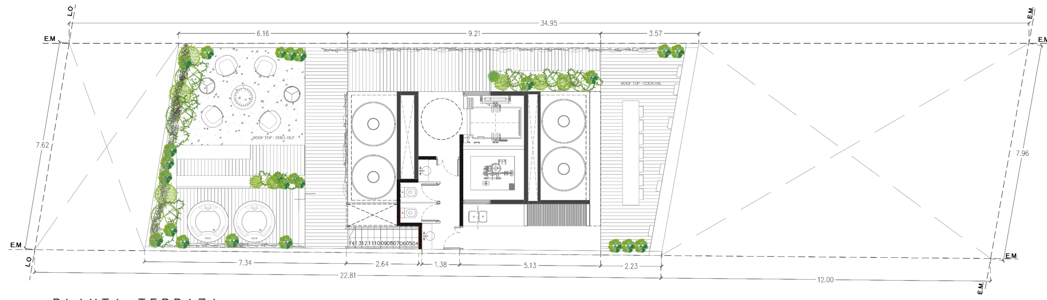
PLANTA TERRAZA
